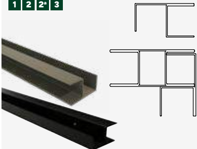
Hoekprofiel t.b.v. hoekpaal Gepoedercoat metaal
